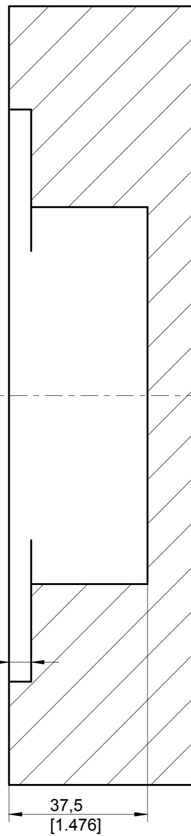
template door panel
