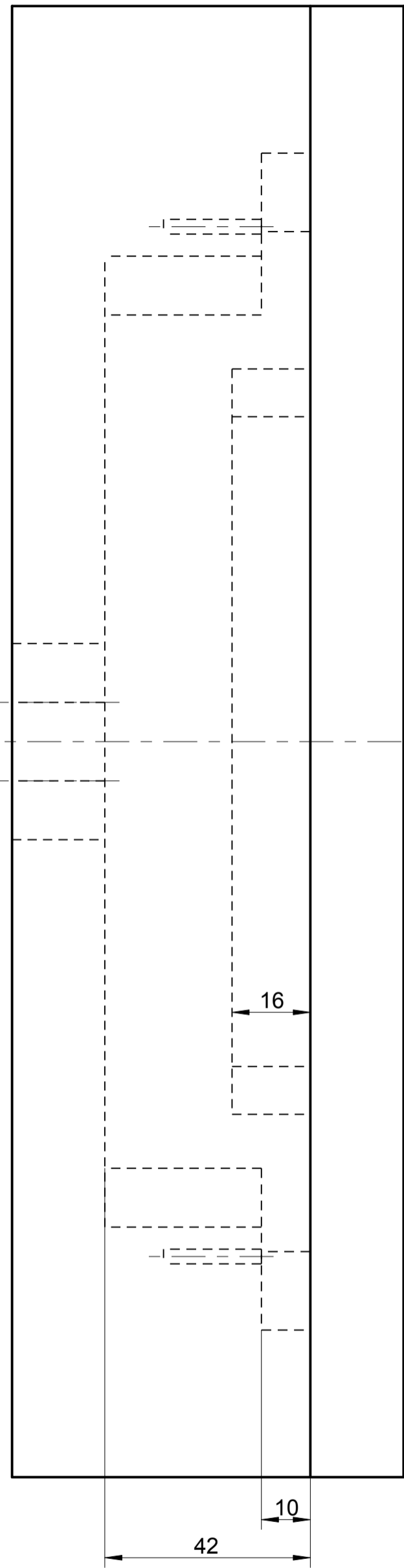
Fräsbild Blockzarge Rahmen
